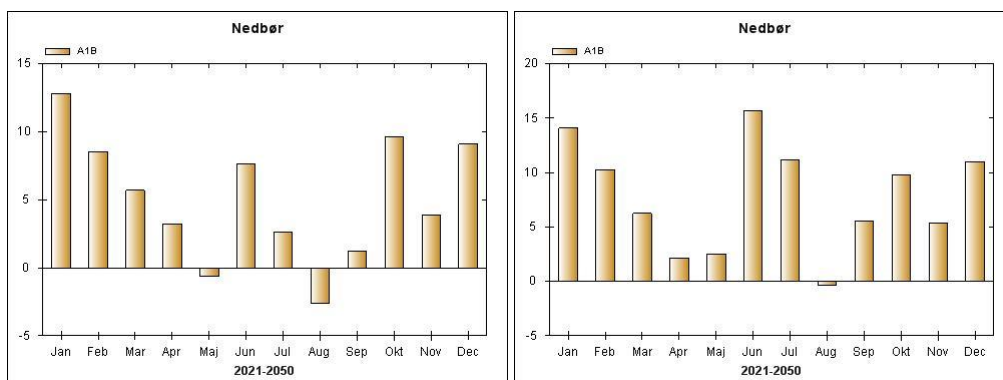
Figur 3.3.4. Relative ændringer i den gennemsnitlige døgngnedbør i en måned i perioden 2021-2050 i A1B scenariet sammenlignet med perioden 1961-1990. Figuren til venstre er Odense og til højre København.
