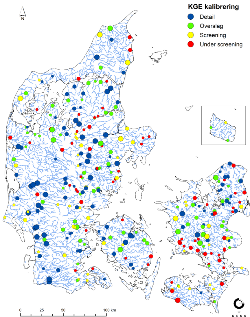
Figur 3: Rumlig fordeling af KGE nøjagtighedsniveauer for alle vandføringsstationer i kalibreringsperioden 2000-2010. Cirklernes størrelse angiver oplands-størrelsen, små cirkler < 100\text{ km}^2 , mellem cirkler mellem 100\text{-}200\text{ km}^2 og store cirkler > 200\text{ km}^2 .
