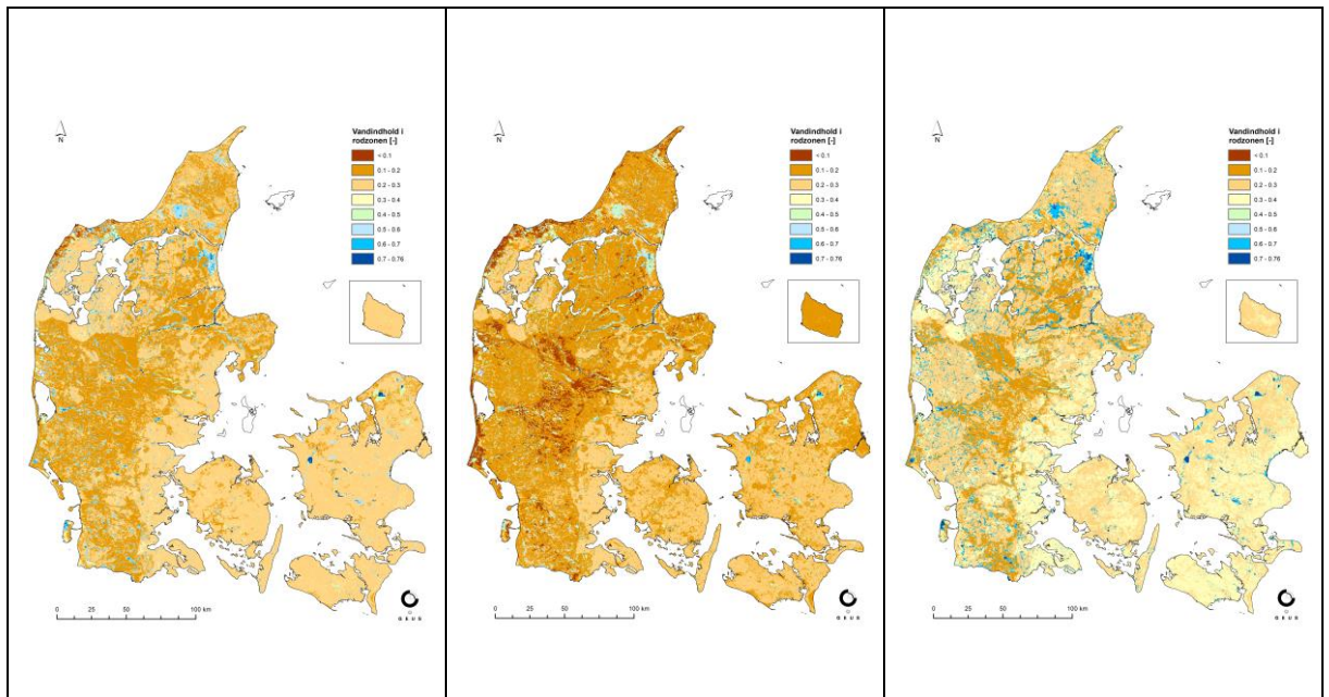
Figur 5. Vandindhold i umættet zone som middel for hele perioden, sommer perioden og vinter perioden 1990 – 2019.
