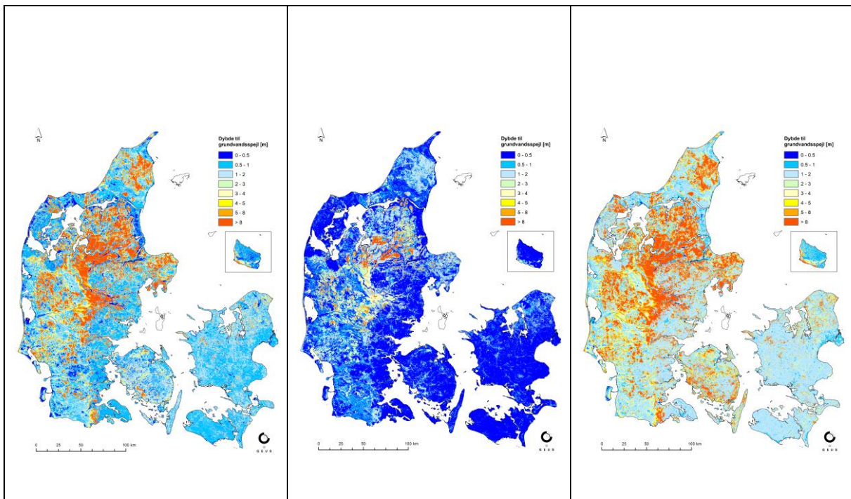
Figur 4. Dybden til terrænnært grundvand, (fra venstre) middel dybde, mindste dybde samt største dybde for perioden 1990 – 2019.
