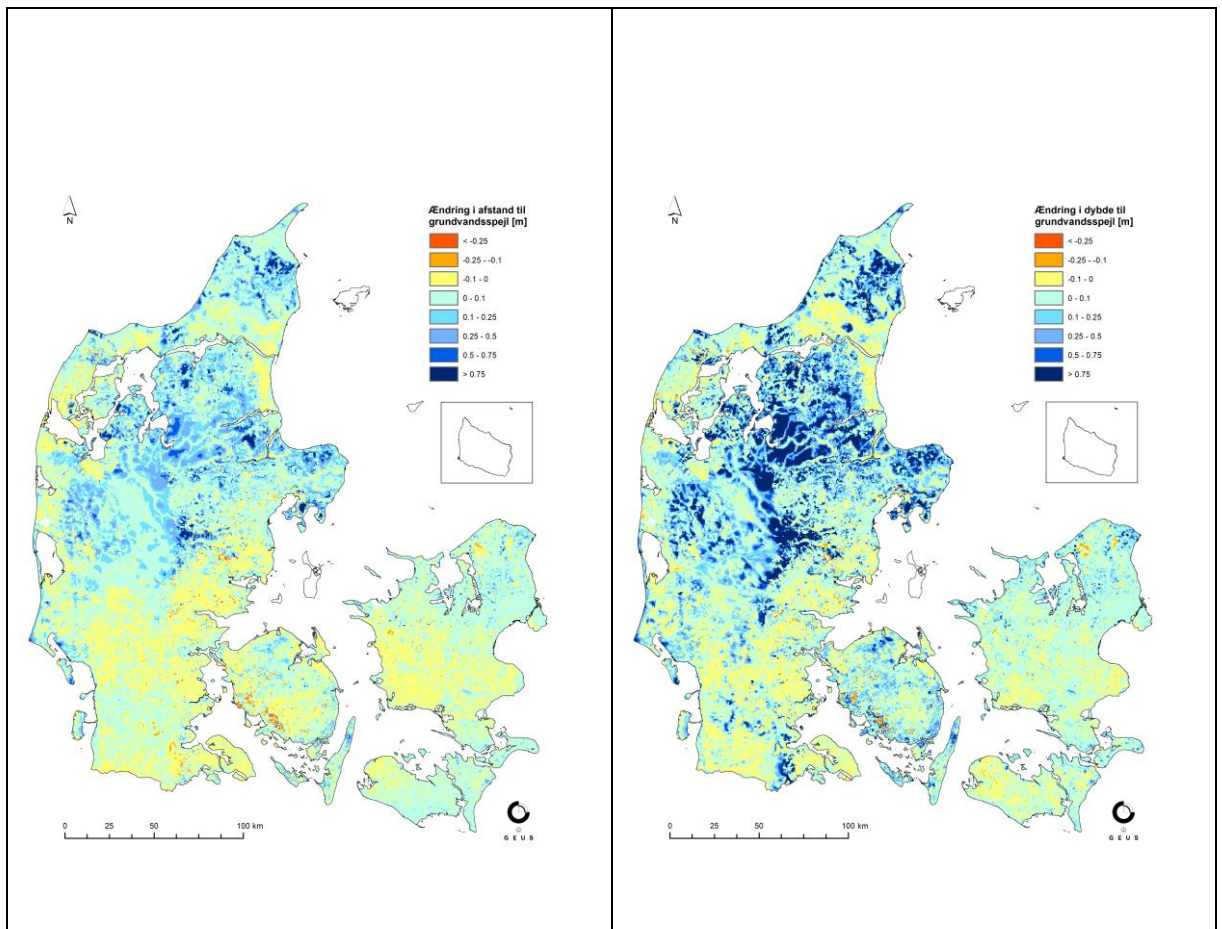
Figur 7. DK-model HIP 500m klimafremskrivning, ændringen i dybden til det terrænnære grundvand, fjern fremtid 2071-2100. Median. RCP4.5 til venstre og RCP8.5 til højre.
