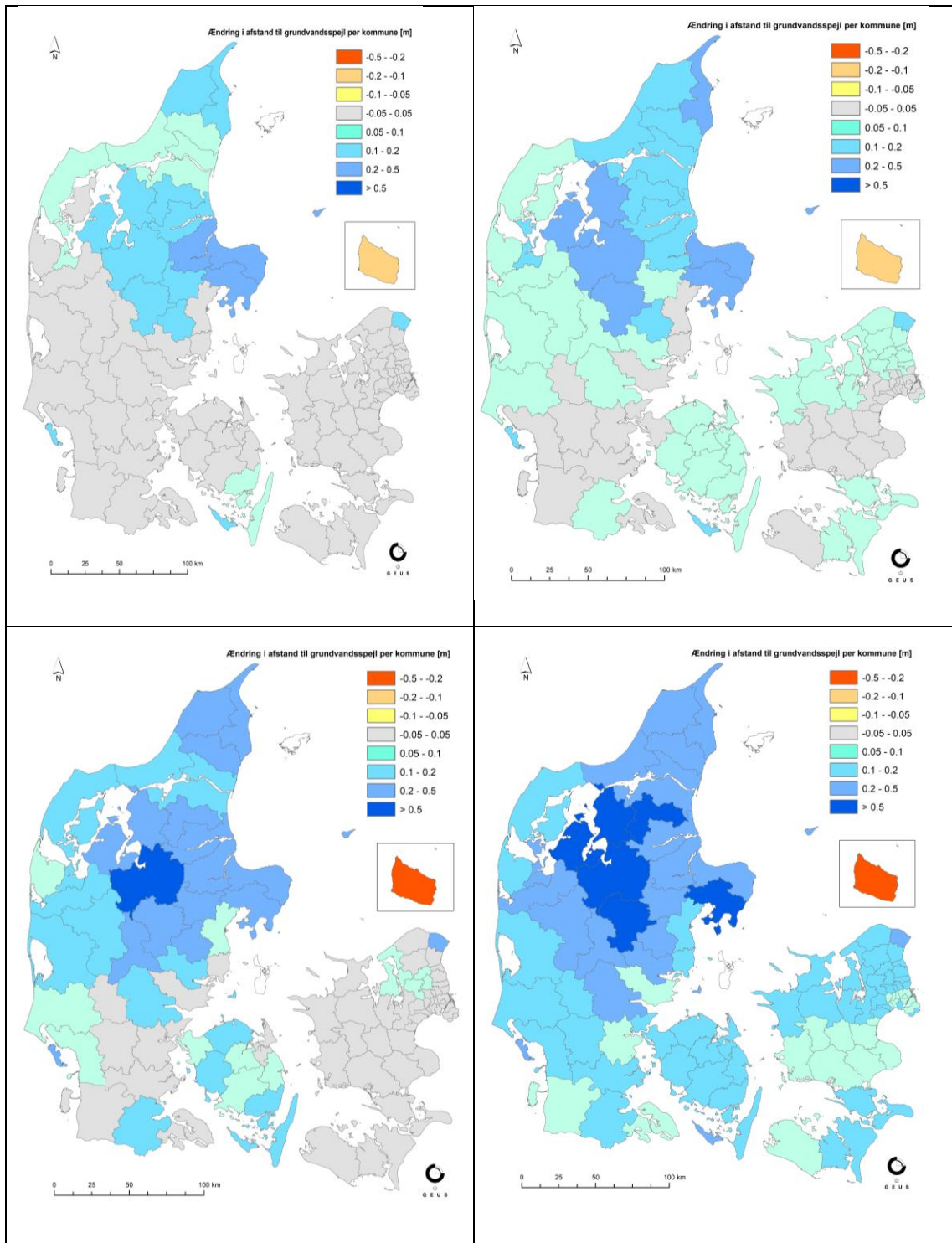
Figur 11: Ændringen i dybden til det terrænnære grundvand per kommune. Fra øverst tv. - RCP4.5 nær fremtid sommer, RCP4.5 nær fremtid vinter, RCP4.5 fjern fremtid sommer, RCP4.5 fjern fremtid vinter, RCP8.5 nær fremtid sommer, RCP8.5 nær fremtid vinter, RCP8.5 fjern fremtid sommer, RCP8.5 fjern fremtid vinter. Bemærk. Granskning har påvist en fejl i processering af klimafremskrivning for Bornholm, genberegning er igangsat og forventes implementeret i løbet af marts 2021.
