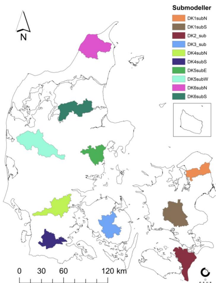
Figur 1: Oversigt af geografisk placering af submodeller.
