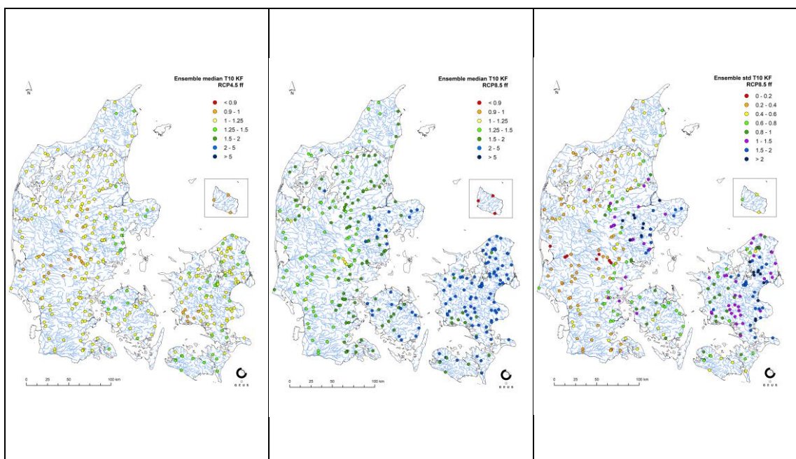
Figur 10: Klimafremskrivning, median på klimafaktor på 10-års maksimal vandføring fjern fremtid, RCP4.5 til venstre og RCP8.5 i midten, standardafvigelsen til RCP8.5 fjern fremtid til højre. Viser kun vandføringsstationer. Bemærk. Granskning har påvist en fejl i processering af klimafremskrivning for Bornholm, genberegning er igangsat og forventes implementeret i løbet af marts 2021.
