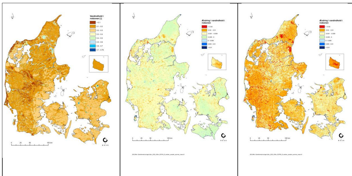
Figur 8: Historisk 100 m sommer middel, ændring i vandindholdet i rodzonen RCP4.5 sommer median fjern fremtid og RCP8.5 sommer median fjern fremtid. ændring i vandindholdet. Bemærk. Granskning har påvist en fejl i processering af klimafremskrivning for Bornholm, genberegning er igangsat og forventes implementeret i løbet af marts 2021.
