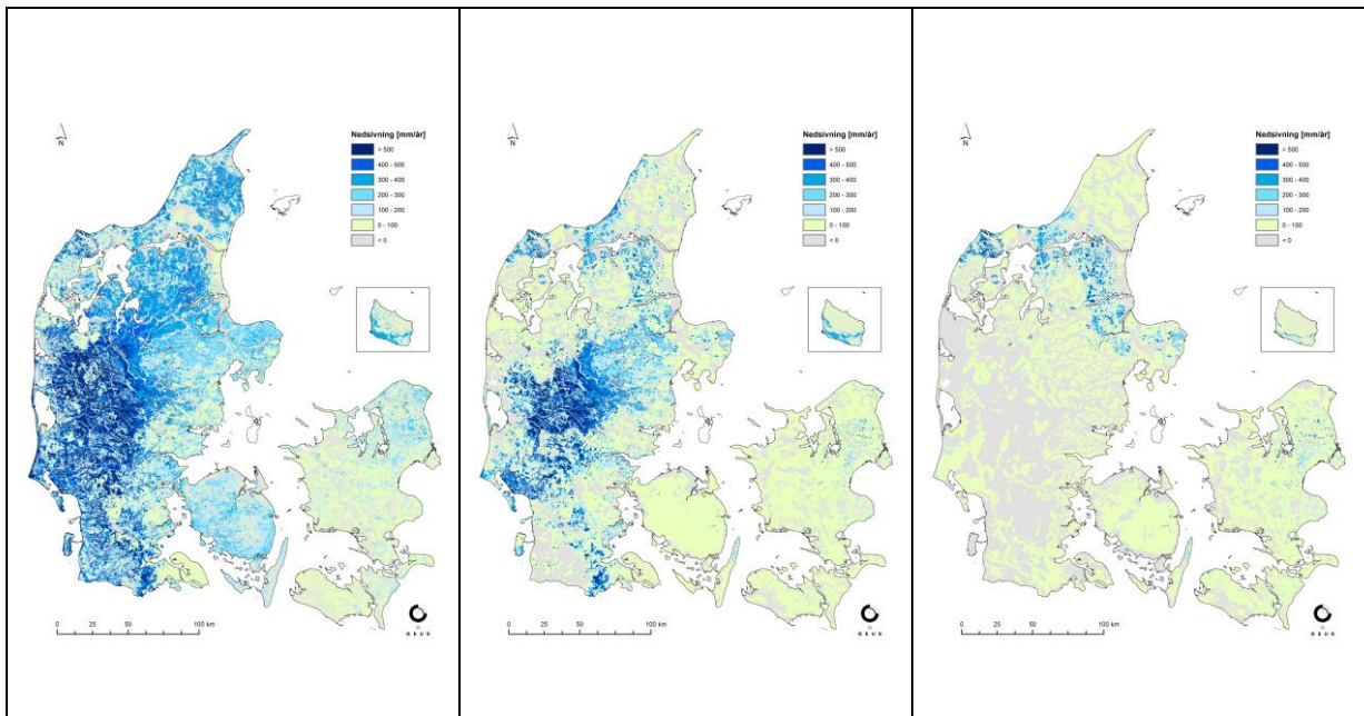
Figur 17. Middelværdi af nedsvivning til magasinlag ks1, ks3, ks4-6 og kalken i perioden 1990 – 2019 (mm/år).
