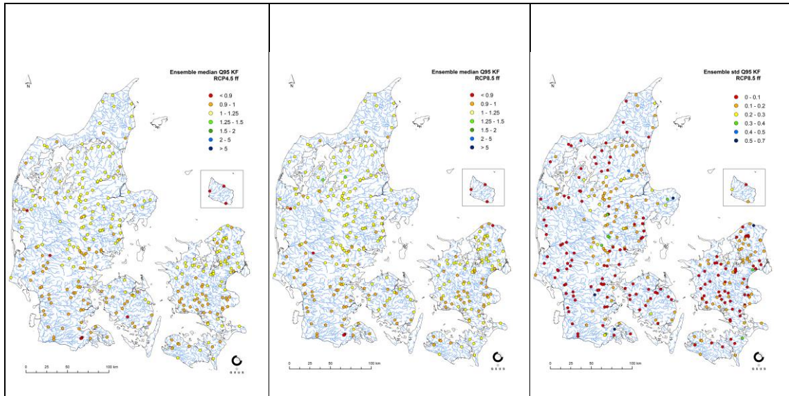
Figur 9: Klimafremskrivning, median på klimafaktor Q95, RCP4.5 til venstre og RCP8.5 til højre. Standardafvigelsen for RCP8.5 fjern fremtid vises th. Viser kun vandføringsstationer.
