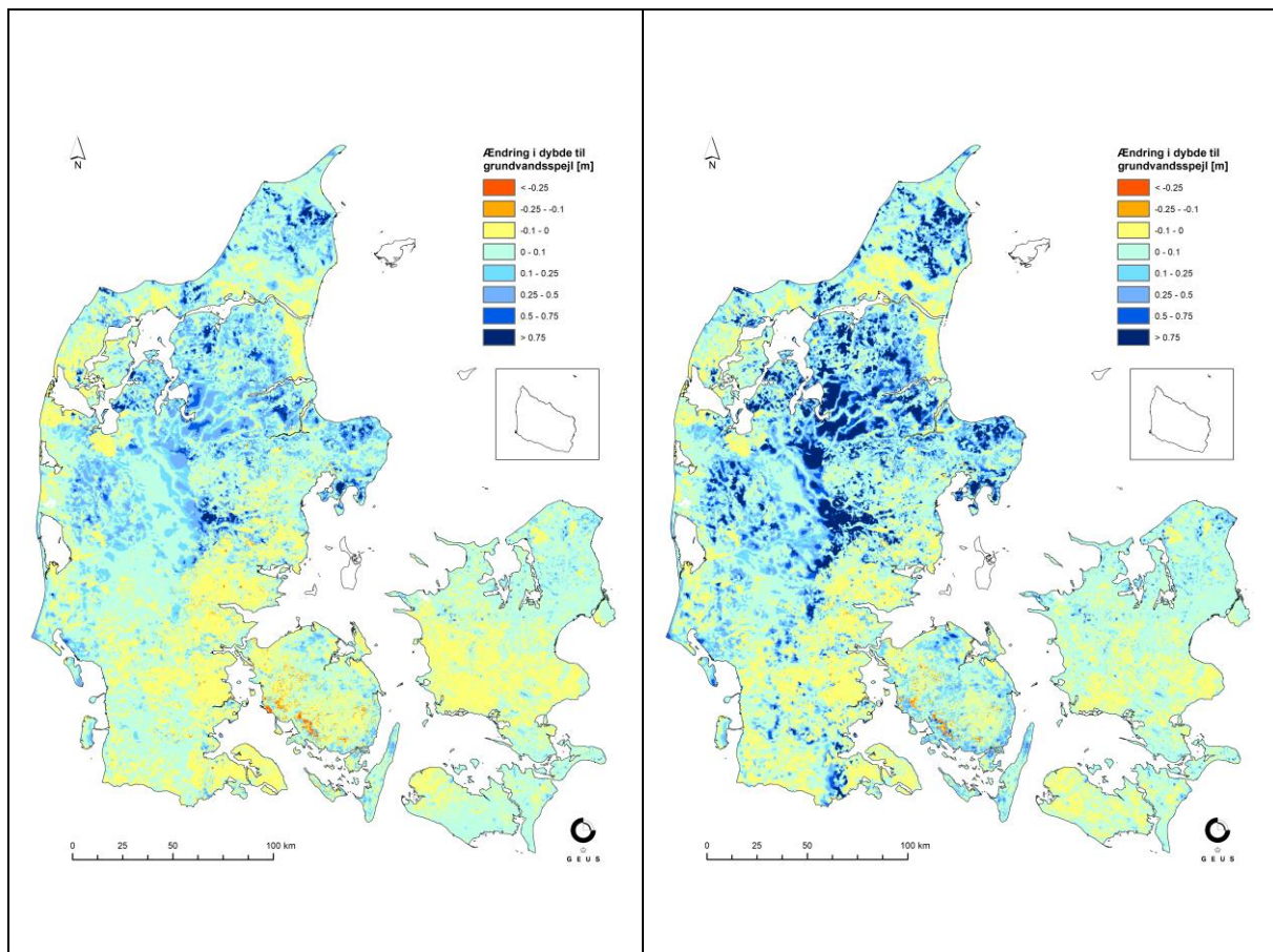
Figur 12. Nedskaleret ændring i dybden til grundvandsspejlet, fjern fremtid. RCP4.5 til venstre og RCP8.5 til højre. Gennemsnit for hele året.
