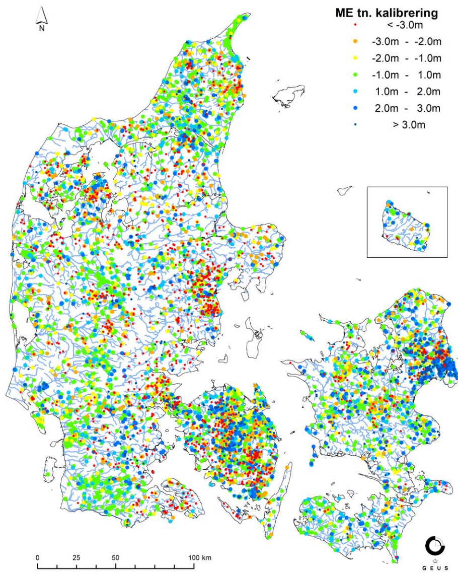
Figur 2: Rumlig fordeling og størrelse af middelfejl (ME) for alle observerede terrænnære trykniveauer i kalibreringsperioden 2000-2010. Symbolrækkefølgen bevæger sig fra grøn (bagerst) til henholdsvis rød og mørkeblå (forrest). Områder med større afvigelser bliver således fremhævet på figuren.
