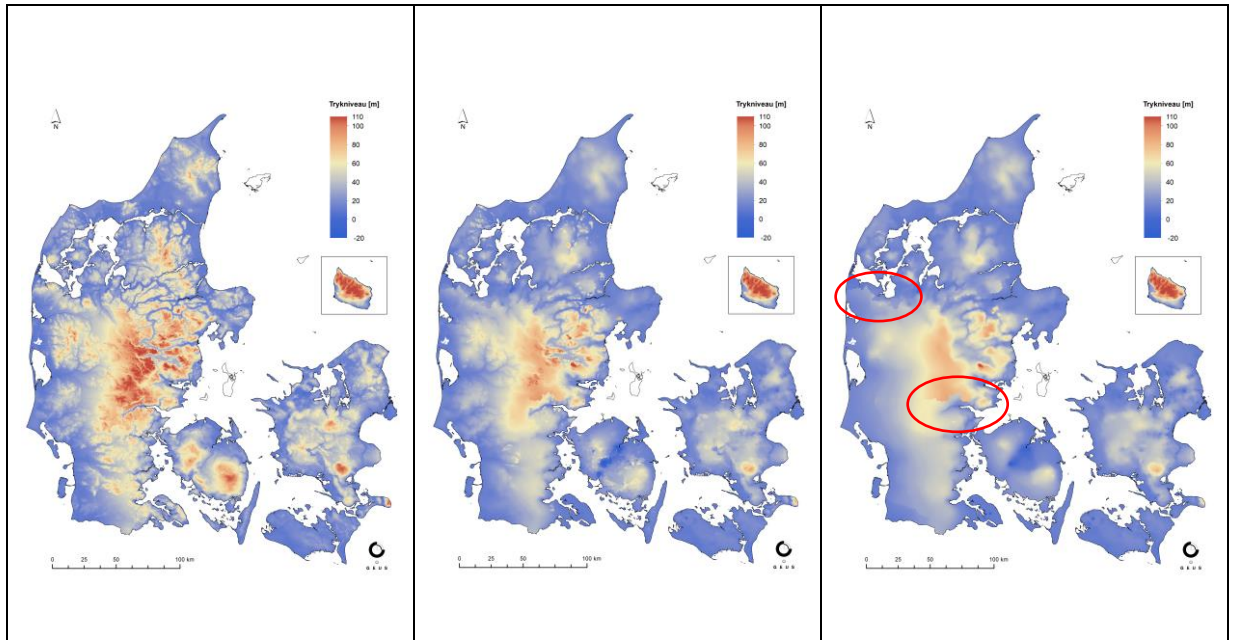
Figur 18. Simuleret middeltrykniveau i perioden 1990 – 2019 for magasinlag, ks1, ks3 og kalken (m DVR).
