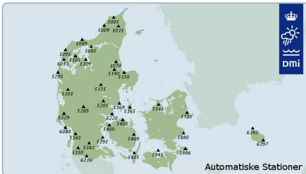
Placering og stationsnumre for de automatiske stationer. Kilde: DMI Teknisk Rapport 12-06.
